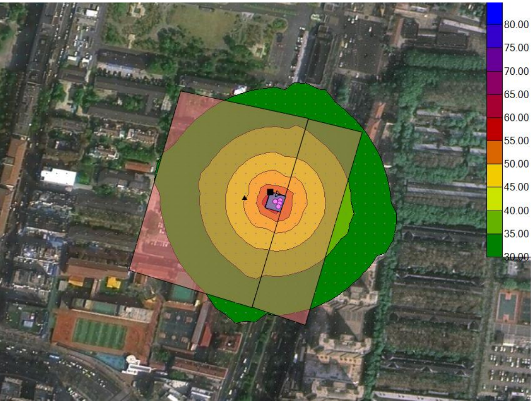
图 4-3 噪声预测贡献值等值线分布图
